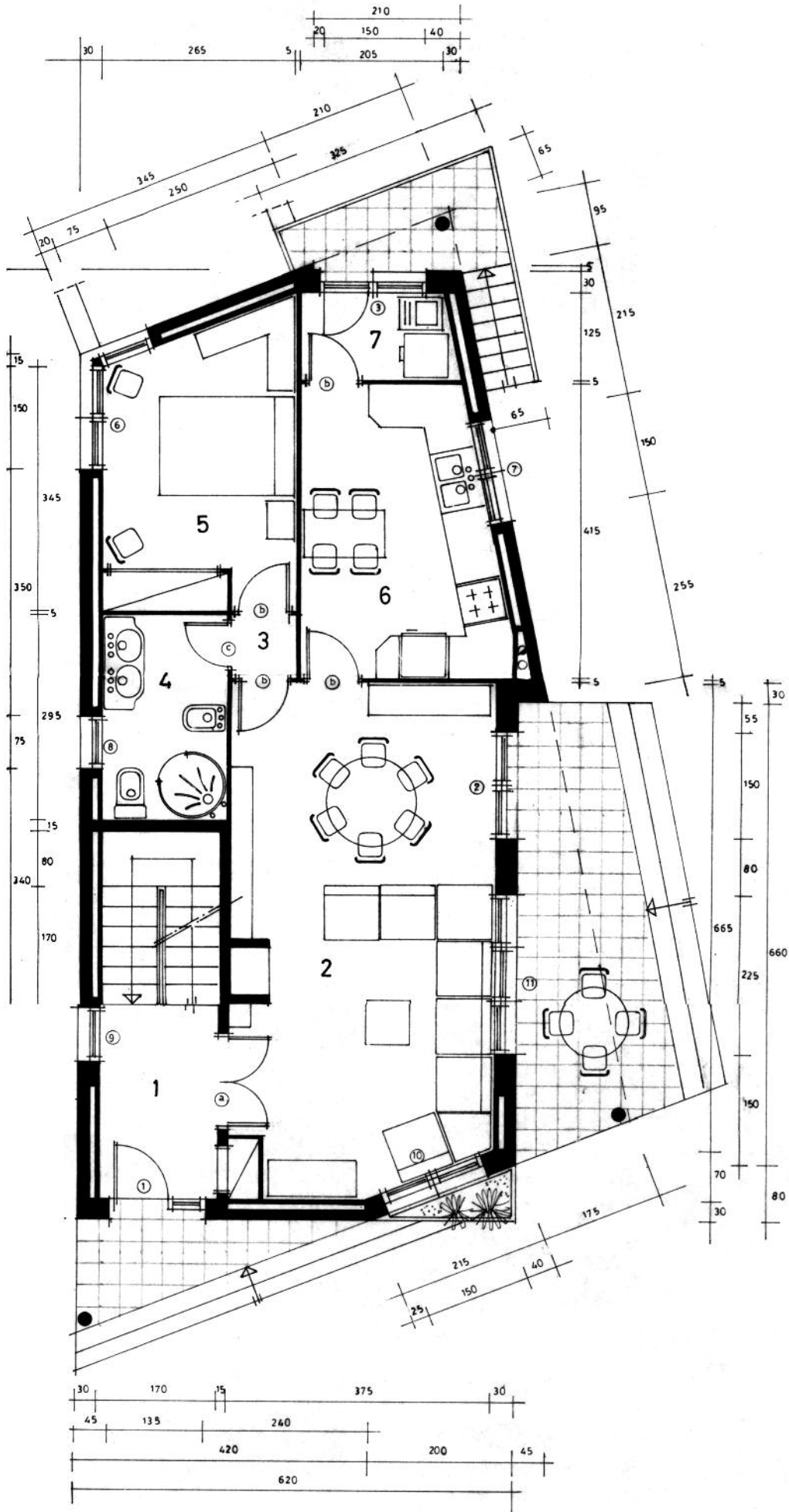
PLANTA BAJA
