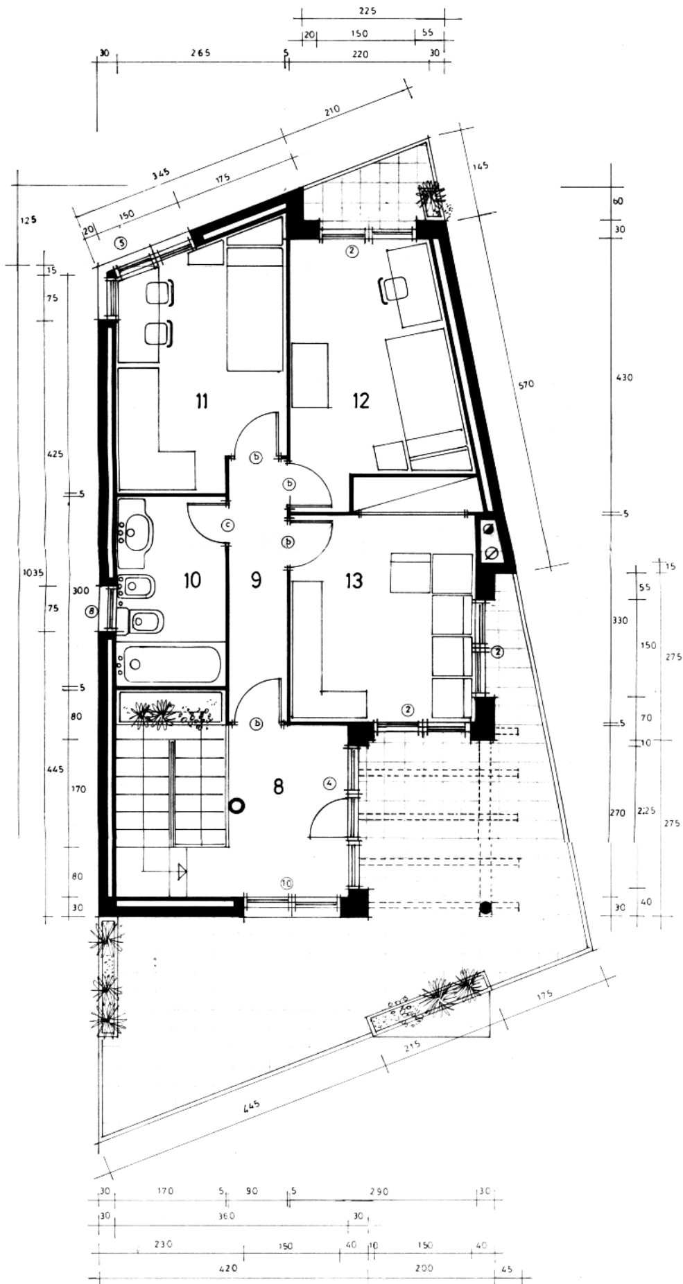
PLANTA PISO
