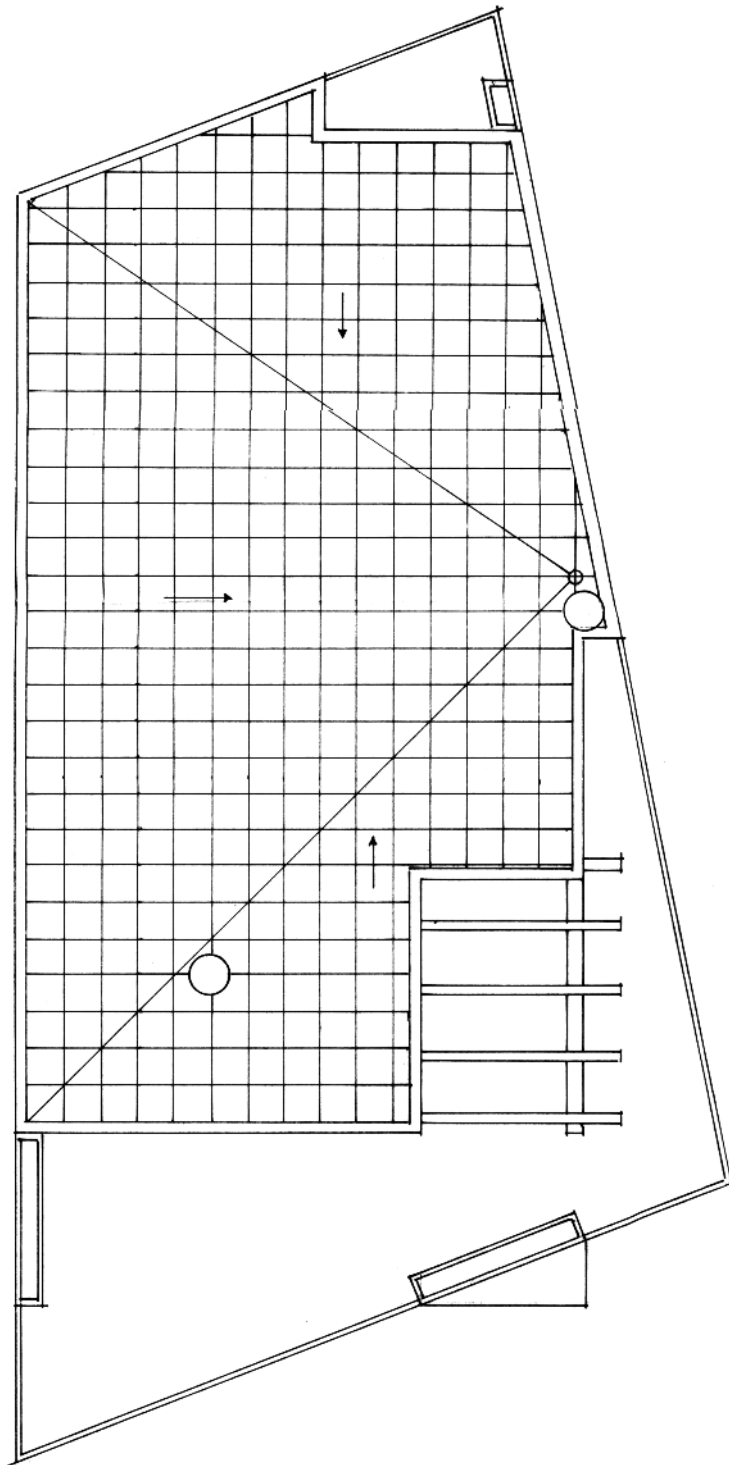
PLANTA CUBIERTA
