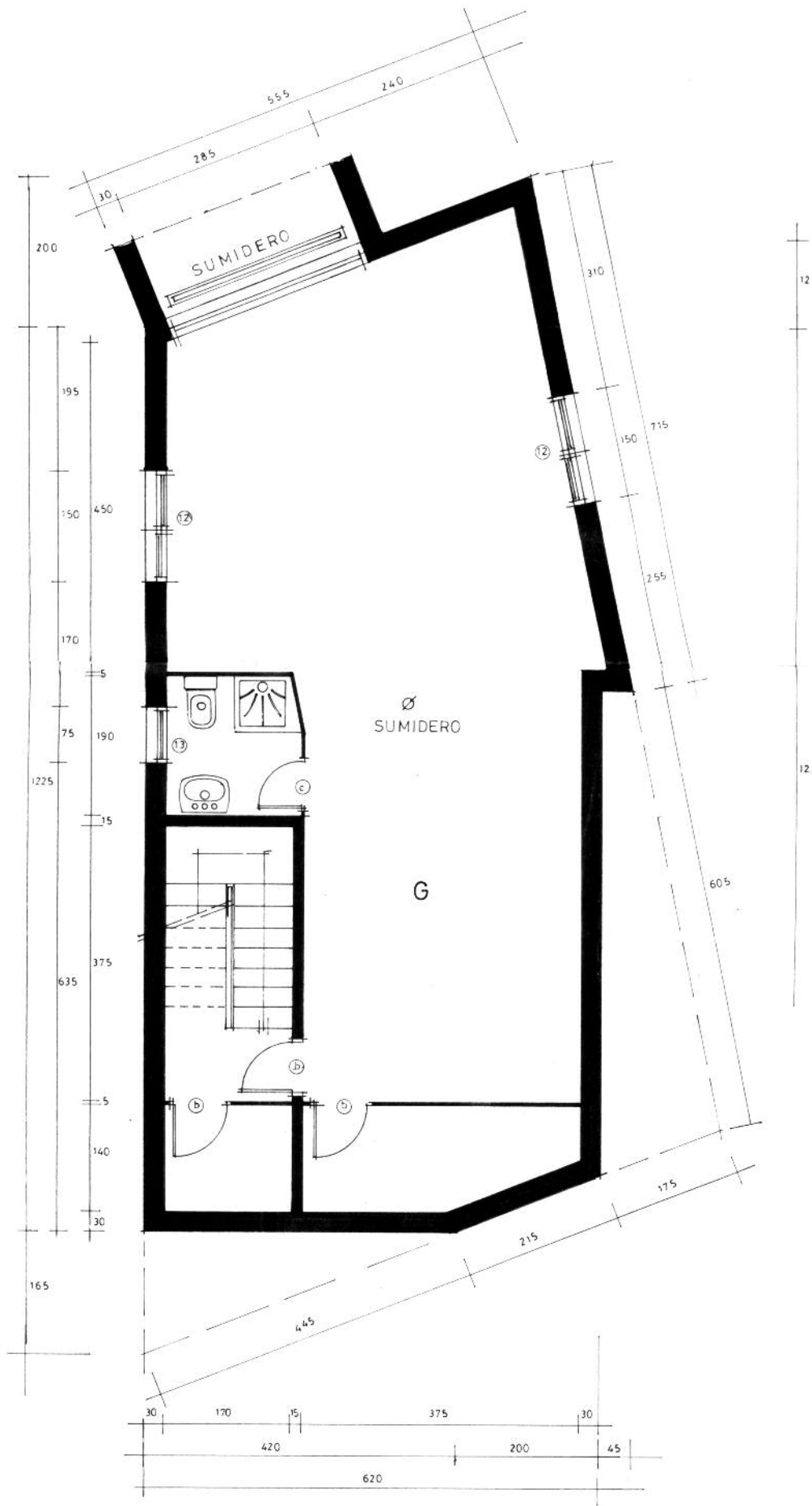
PLANTA SOTANO
